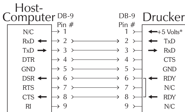
DB9-Buchsenstecker/DB9-Stecker
