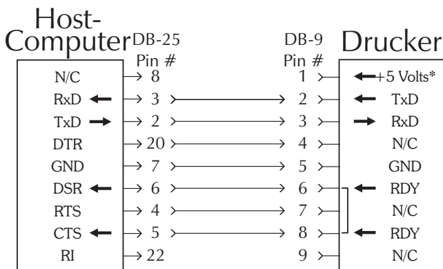
DB25-Buchsenstecker/DB9-Stecker
